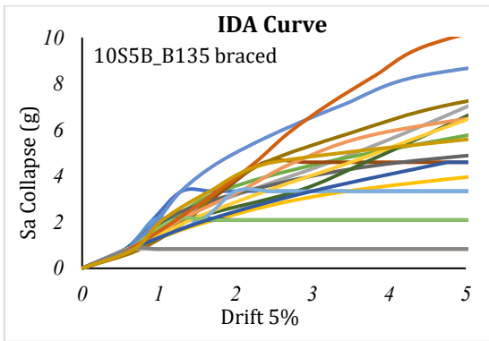
شکل ۲۵- نمودار تحلیل دینامیکی افزایشدهنده قاب پنج دهانه با دهانه‌های ۲ و ۴ مهاربندی
