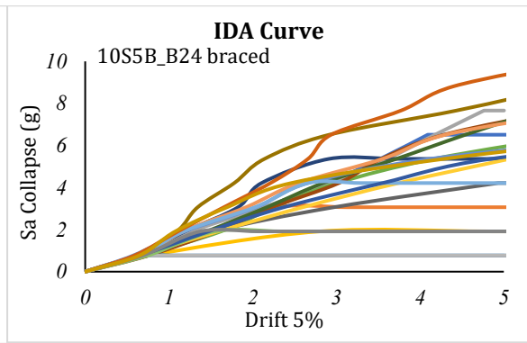
شکل ۲۴- نمودار تحلیل دینامیکی افزایشدهنده قاب پنج دهانه با دهانه‌های ۱، ۳ و ۵ مهاربندی
