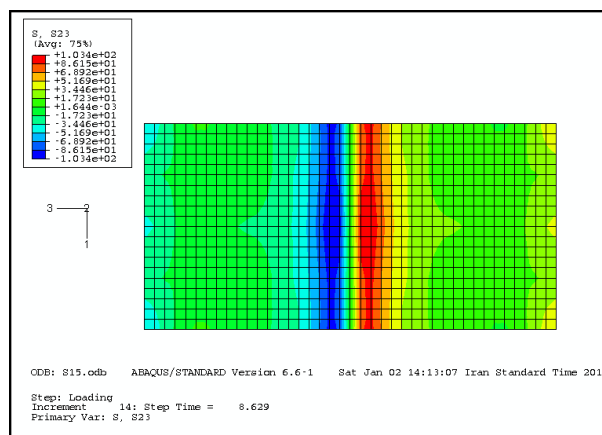
شکل (۹): نمایش تنشهای برشی داخل لایه چسب اتصال دهنده فولاد و CFRP
