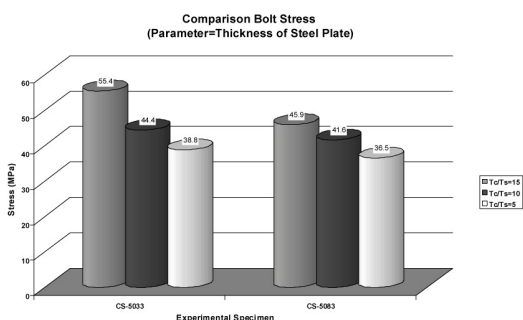
شکل (۱۱): مقایسه تنش ماگزیمم برش گیر بر اساس تغییر ضخامت صفحه فولادی
