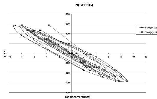
شکل (۱): مقایسه نتایج بار - جابجایی تحلیل عددی و مدل آزمایشگاهی برای نمونه SSW
