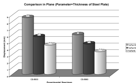
شکل (۷): مقایسه تغییر شکل‌های داخل صفحه بر اساس تغییر ضخامت صفحه فولادی
