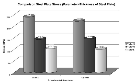
شکل (۹): مقایسه تنش ماگزیمم صفحه فولادی بر اساس تغییر ضخامت صفحه فولادی
