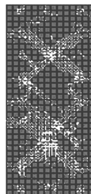
شکل (۶) : مقایسه ترکهای ناشی از بارگذاری مدل آزمایشگاهی با تحلیل عددی ( نمونه CS-5-3x8 )
