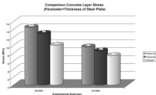
شکل (۱۰): مقایسه تنش ماگزیمم صفحه بتنی بر اساس تغییر ضخامت صفحه فولادی
