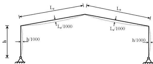
شکل (۱۵): الگوی نقص شکم‌دادگی در قاب شیب‌دار
