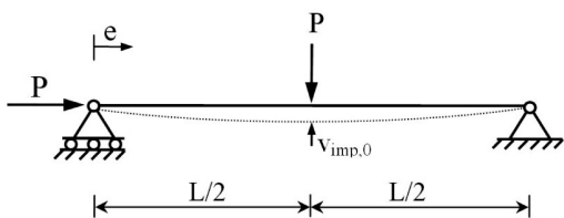
شکل (۸): ستون لاغر دو سر مفصل با نقص انحنای نخستین
