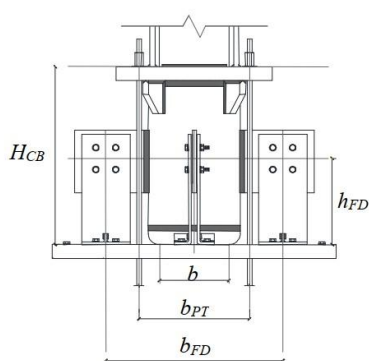
شکل ۷- پارامترهای هندسی پایه ستون گهواره‌ای [۱۰]
