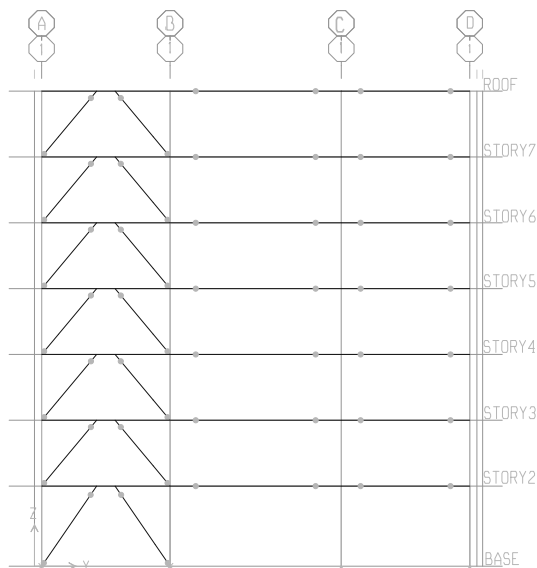
ب) نمای سازه RL-EBRB
