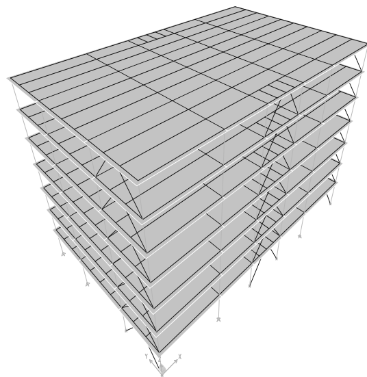
الف) مدل سه بعدی
