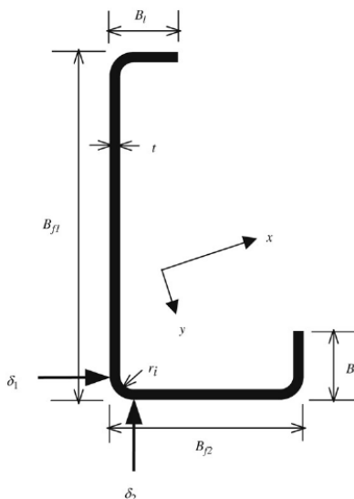
شکل ۱- مقطع نبشی مورد آزمایش با بال‌های نامساوی [۵]
