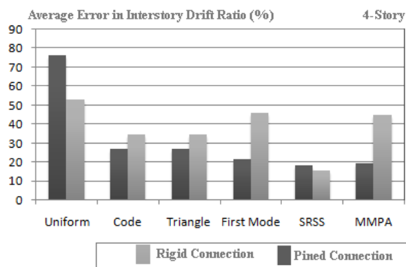
شکل ۵- خطای پارامتر لرزه‌ای جابه‌جایی بین طبقه‌ای به صورت درصدی از ارتفاع طبقه در مدل چهار طبقه
