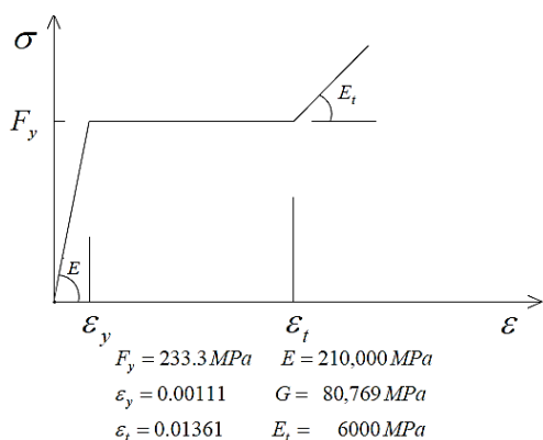
شکل ۱- منحنی تنش کرنش فولاد
