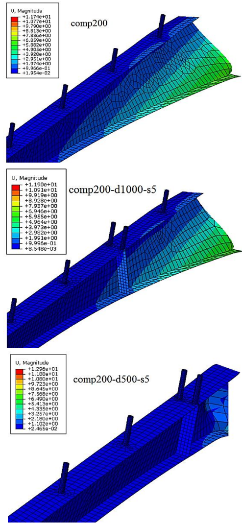
شکل ۹- کانتورهای تغییر شکل جانبی در تیر با موقعیت قرارگیری متفاوت سخت‌کننده
