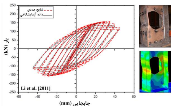
ب) نمونه SP2 [۲۵]
