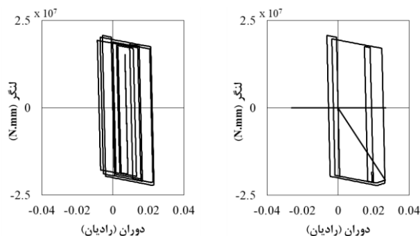
قاب با اتصالات خمشی متداول قاب دارای بازشو در جان تیر الف) قاب خمشی دو دهانه [۳۰] تحت رکورد دوزجه با شتاب طیفی
