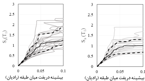
قاب با اتصالات خمشی متداول / قاب دارای بازشو در جان تیر
