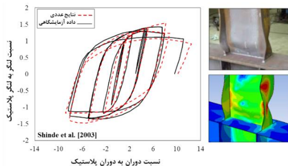
الف) نمونه SP1 [۲۴]
